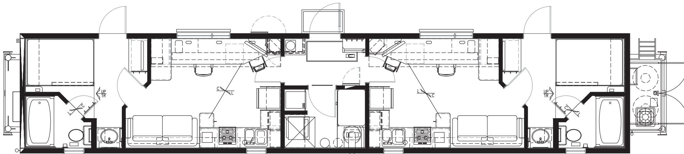
12' x 60' (skid) WELLSITE "ENG./ENG."
